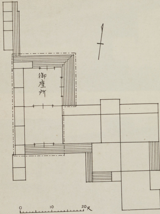
明治天皇鶴御小休所御座所建物現狀平面圖 (點線部分が移築の建物)
