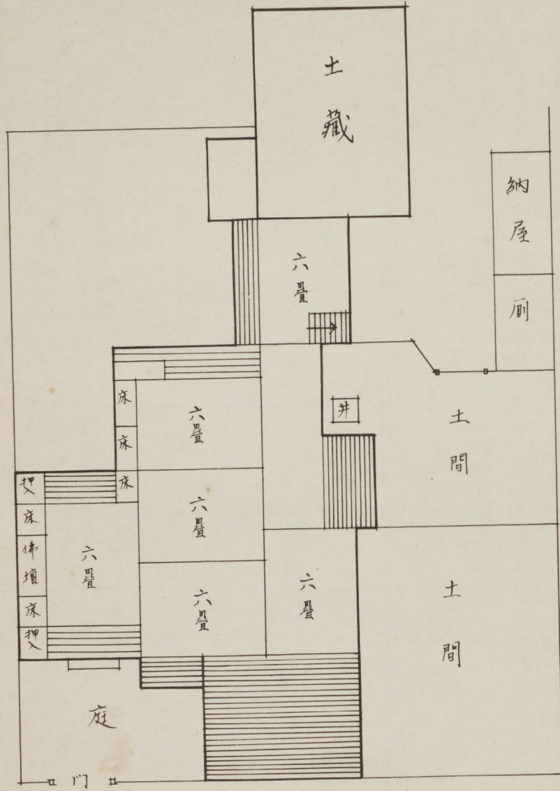
明治天皇鶴御小休所(元大西邸現三木邸)現狀平面圖
