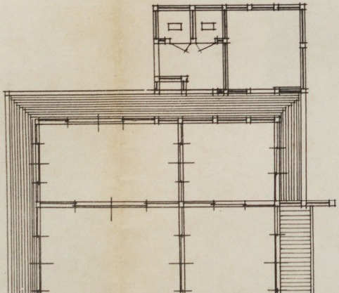
明治天皇加古川行在所山脇邸現狀平面圖
