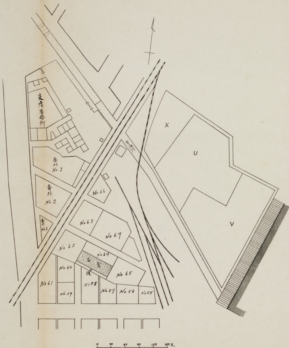
神戶御用邸 陸(三菱倉庫株式會社神戶支店所有地)實測平面圖
