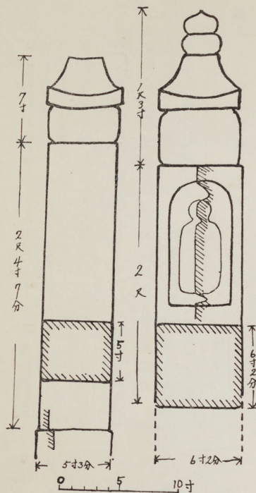
第廿圖 諭鶴羽神社町石實測圖 (左圖は建武銘のもの、右圖は十六丁目附近にあるもの)
