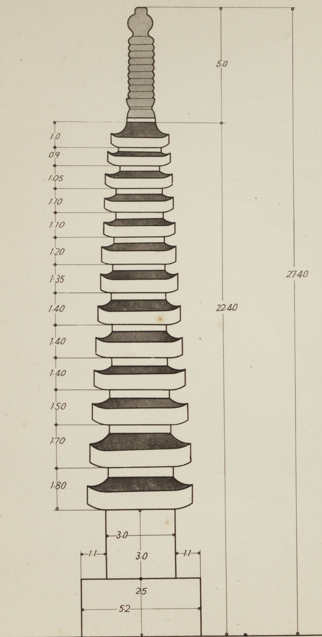
清盛塚實測圖
