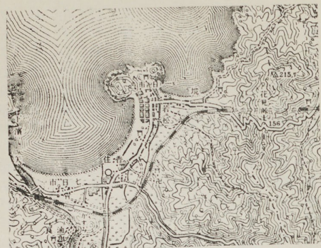
第五廿五圖 香住町附近地圖 (陸地測量部五萬分一地圖)
