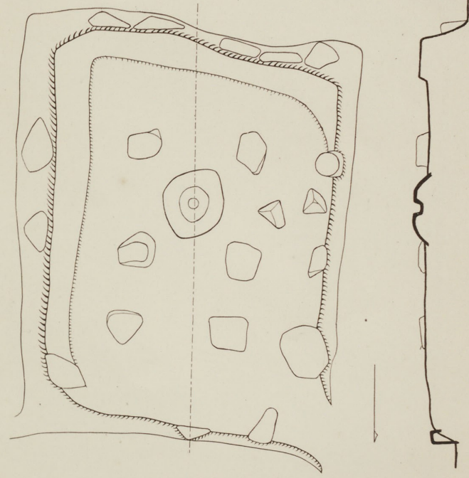
塔址實測圖 (式部測圖)
